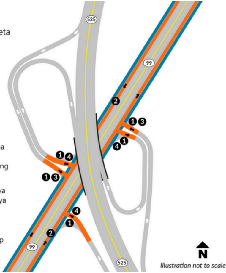
Plan view ng palitan ng daan ng SR 99 at SR 525 na may mga rampa na muling inayos na tumutugma sa SR 99 sa halos sulok na tirik, idinagdag na linya ng pag-access sa negosyo at sasakyang pampubliko, idinagdag na mga daanan para sa paglalakad at pagbibisikleta, at nakataas na tawiran na may mga hudyat sa buong palitan ng daan.
