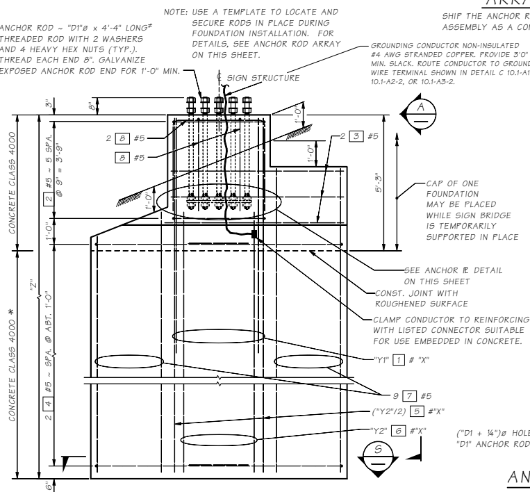
ELEVATION
