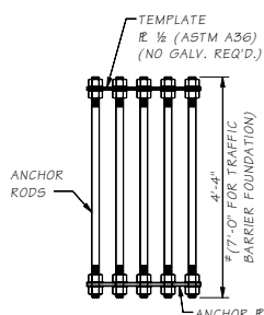
ANCHOR ROD ARRAY
