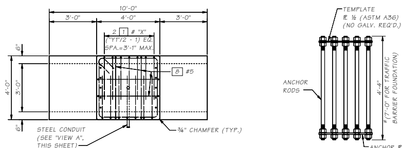
ANCHOR ROD ARRAY
