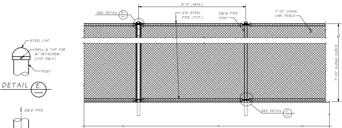
ELEVATION
