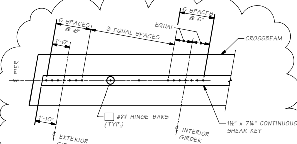
HINGE BAR PLAN
