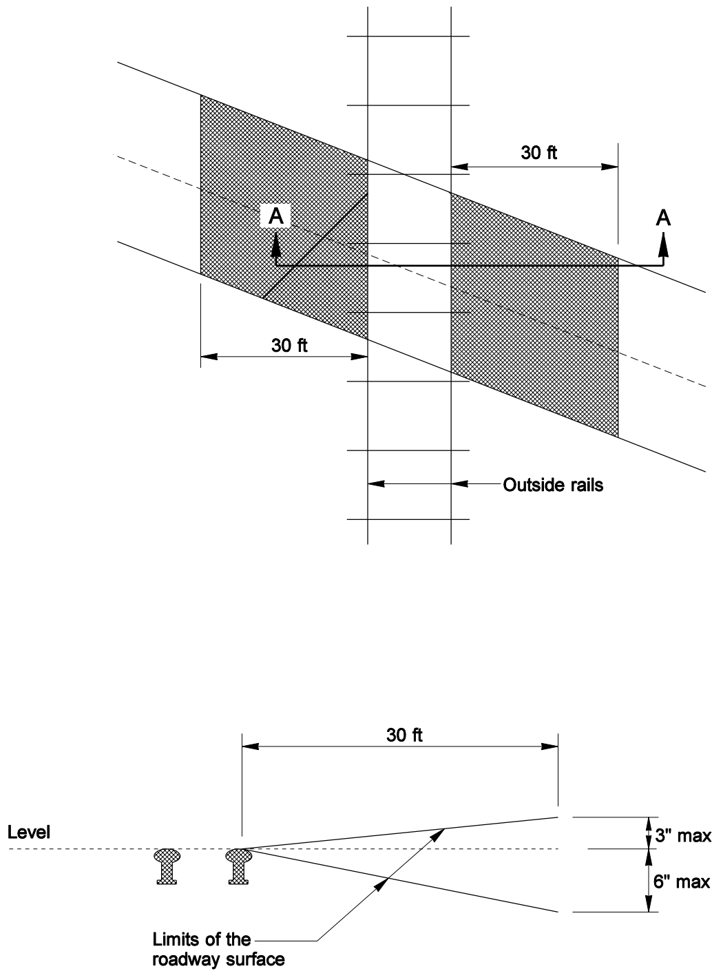
Detail A-A
