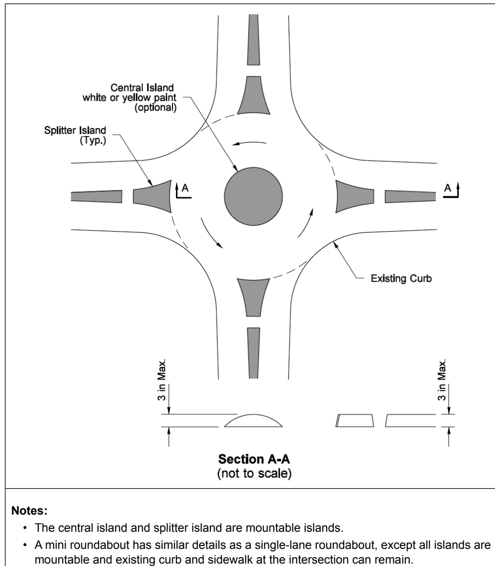
Mini Roundabout Exhibit 1320-4
